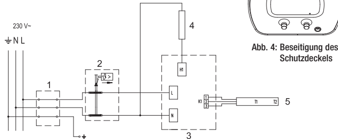
Abb. 5: Elektroschaltbild
