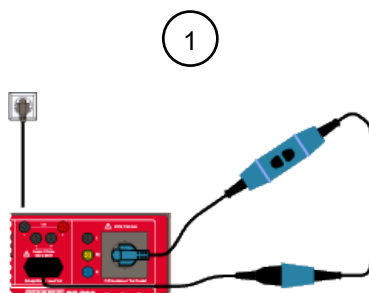
Abb. 27: PRCD prüfen (Anschlussschema)
