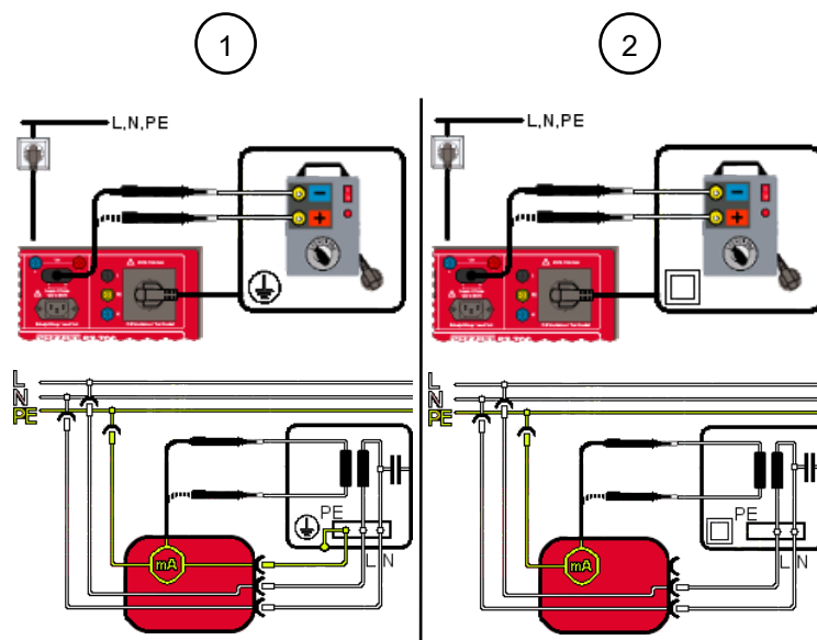
Abb. 26: Berührungsstrom Schweißstromkreis prüfen (Anschlussschema, Stromlaufplan)
