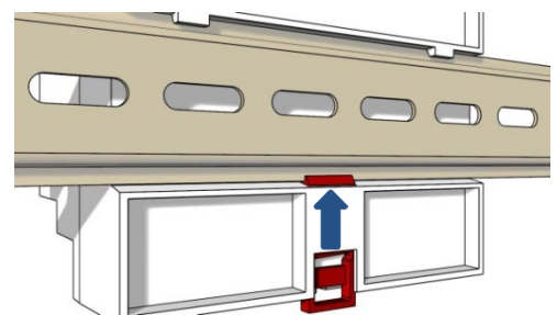
Abb. 3: Einrasten
