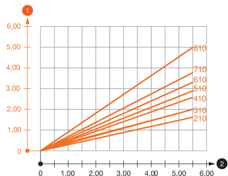
Belastungsdiagramm Ausleger Typ AS 55
