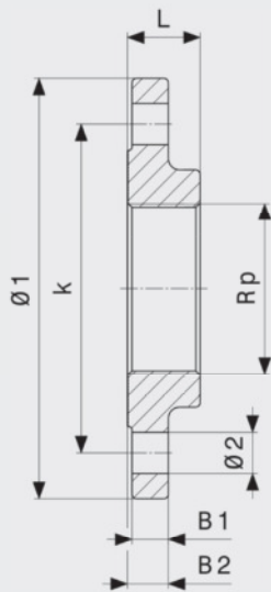
Sanpress XL-Flansch, PN 16 - Rotguss oder Siliziumbronze Modell 2259.2XL
