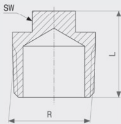
Stopfen - Rotguss oder Siliziumbronze Modell 3291
