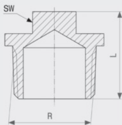
Stopfen - Rotguss oder Siliziumbronze Modell 3290
