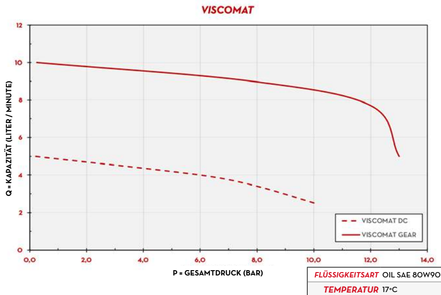
ZAHNRADPUMPE
