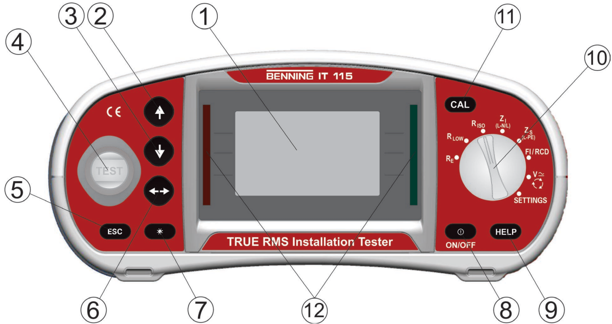
Abbildung 3.1: Vorderseite IT 115
