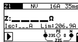
Abbildung 5.26: Leitungsimpedanz
