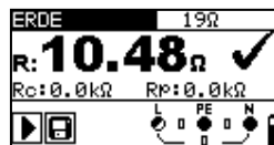
Abbildung 5.35: Beispiel Erdungswiderstandsmessung
