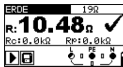
Abbildung 5.35: Beispiel Erdungswiderstandsmessung
