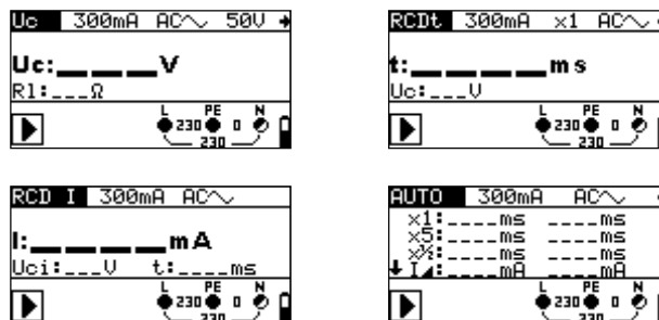
Abbildung 5.16: FI/RCD-Prüfungen
