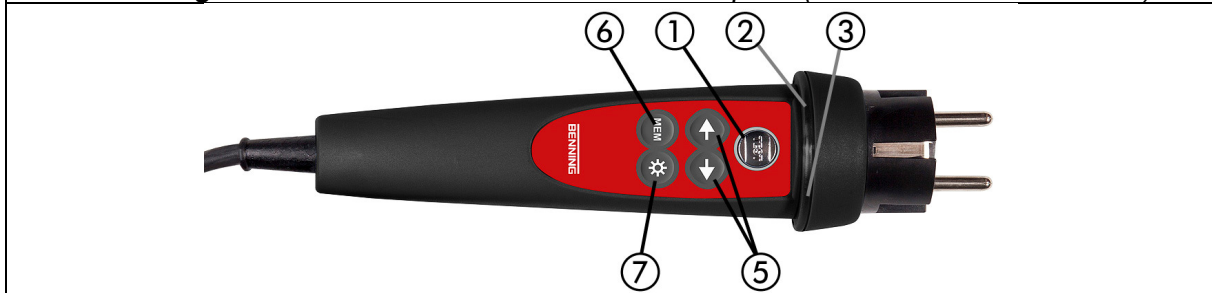
Abbildung C.2: Vorderseite des optionalen Commander-Prüfsteckers für Schutzkontaktsteckdose (schaltbar mit TEST-Taste) (044149)
