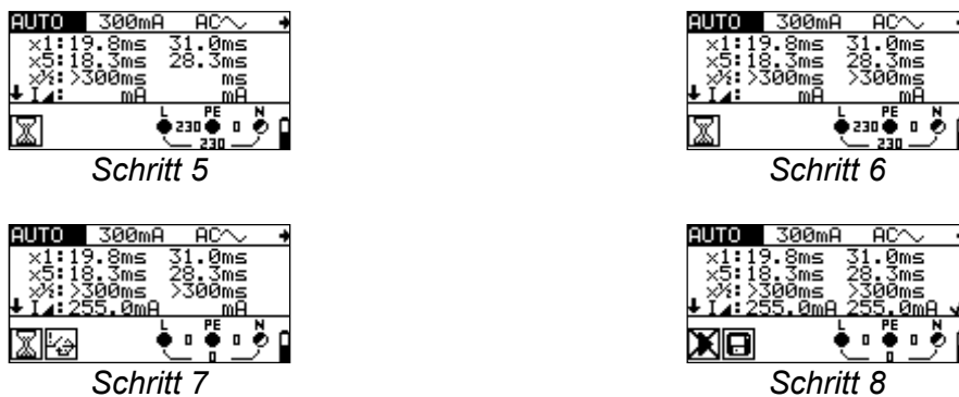
Abbildung 5.21: Prüfschritte der Automatikprüfung
