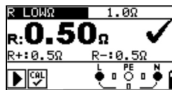
Abbildung 5.10: Beispiel Niederohmmessung R LOWΩ
