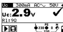
Abbildung 5.18: Beispiel Berührungsspannungsmessung
