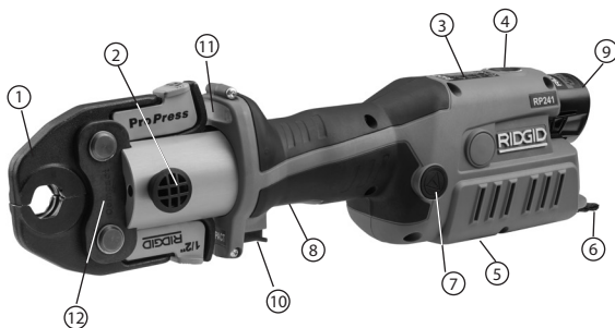
Kuva 2 – RIDGID RP 241 Puristustyökälu ja Compact-sarjan leuka
