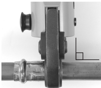
Obrázok 8 – Čeluste usporiadané kolmo na tvarovku
