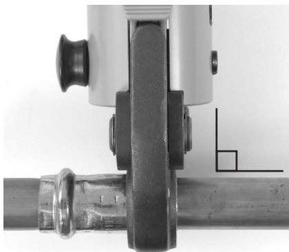
8-сурет – Фитингпен бір деңгейдегі қармауыштар
