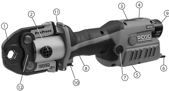
Obrázok 2 – Lisovačka RIDGID RP 241 a čeľusť kompaktnej série
