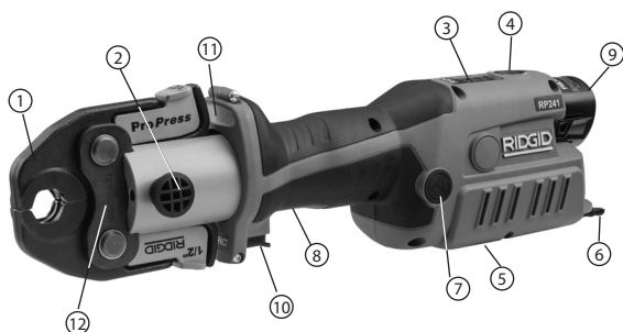
Rysunek 2 – Zagniataarka RIDGID RP 241 i szczęka serii Compact
