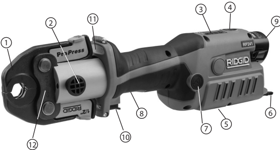
Şekil 2 – RIDGID RP 241 Pres Aleti ve Compact Serisi Çene
