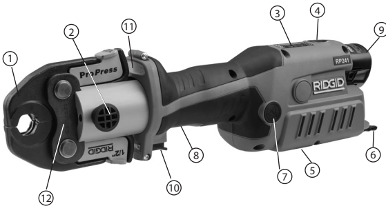
Figuur 2 – RIDGID RP 241 Perswerktuig met bekken van de Compact-reeks
