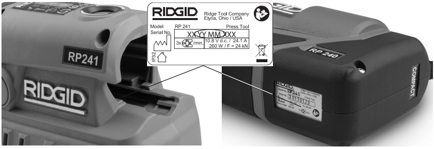
Şekil 3 – Makine Seri Numarası - Daire içindeki rakamlar üretim yılını ve ayını gösterir. (YY = yıl, AA = ay).
