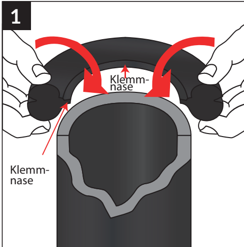
1. Nase in Pfeilrichtung ausdrehen.
