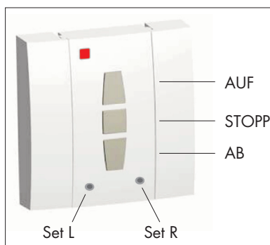
Abb.: Sender, Art. 135000, mit Erklärung der Tastenfunktionen
