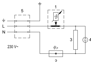
Schéma du couplage électrique
