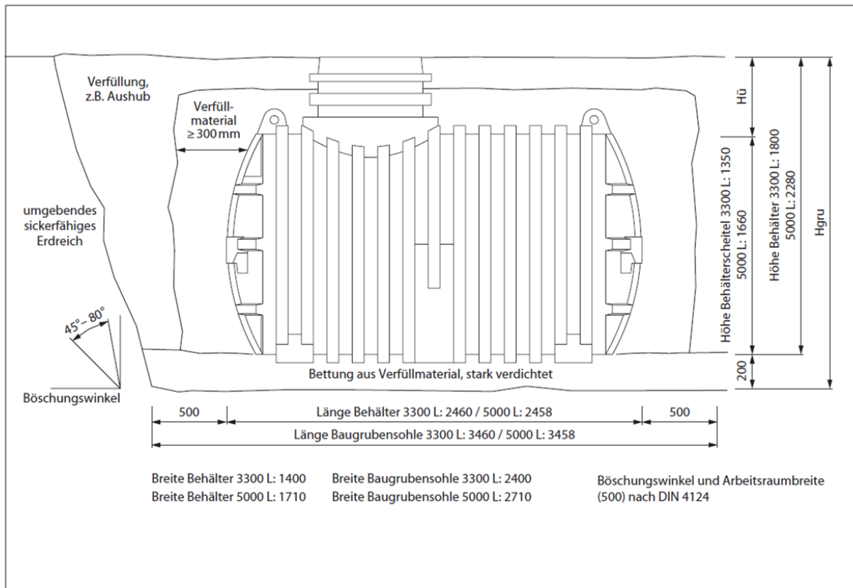
Abbildung 2: Einbaugrößen
