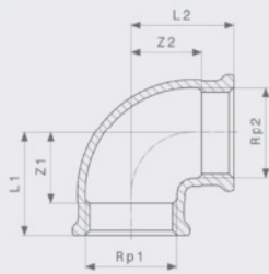
Bogen 90° - Rotguss oder Siliziumbronze Modell 3090
