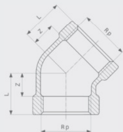
Bogen 45° - Rotguss oder Siliziumbronze Modell 3120
