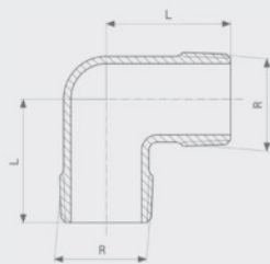
Winkel 90° - Rotguss oder Siliziumbronze Modell 3091
