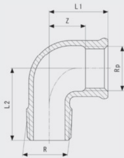
Bogen 90° - Rotguss oder Siliziumbronze Modell 3092
