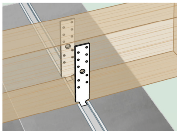
Anwendungsbeispiel SXPA in Halfenschiene
