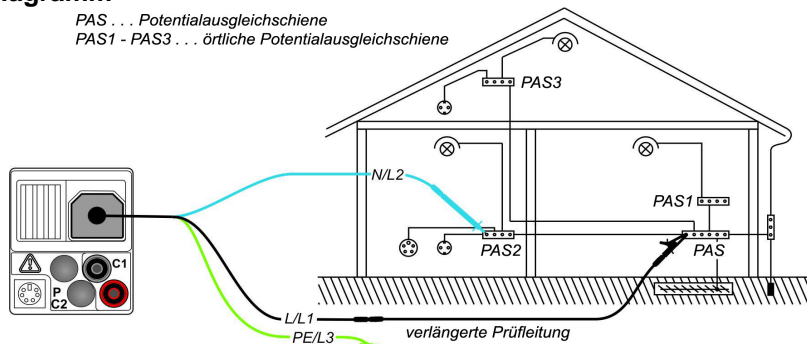
Anschluss der 3-Leiter-Prüfleitung und der optionalen Messleitung BENNING TA 5 (044039)
