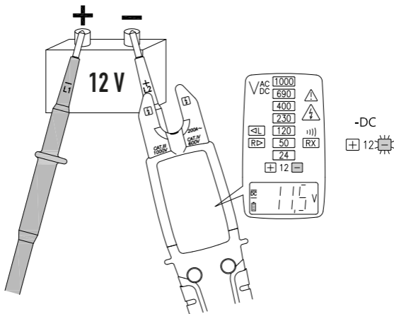
Bild 3: Gleichspannungsmessung Fig. 3: Direct voltage measurement Fig. 3: Mesure de tension continue Obr. 3: Měření stejnosměrného napětí Fig. 3: Medición de tensión continua Εικόνα 3: Μέτρηση συνεχούς τάσης
