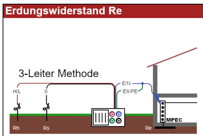
Bild 5.48: 3-Leiter-Anschlussschema
