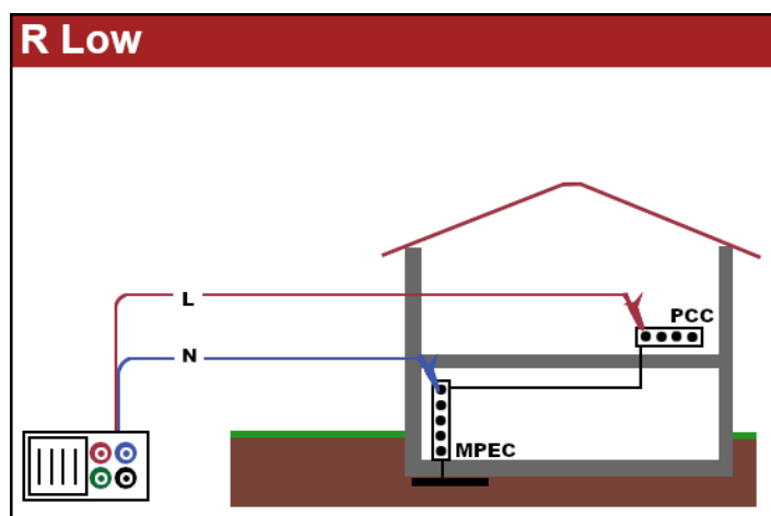
Bild 5.6: kurzgeschlossene Messleitungen
