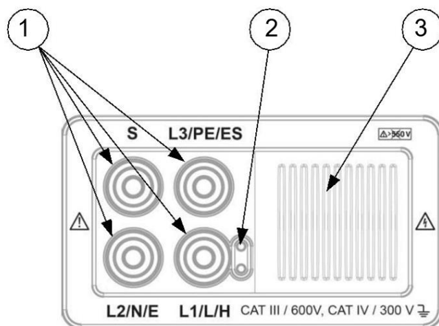
Bild 3.2: Anschlussplatte
