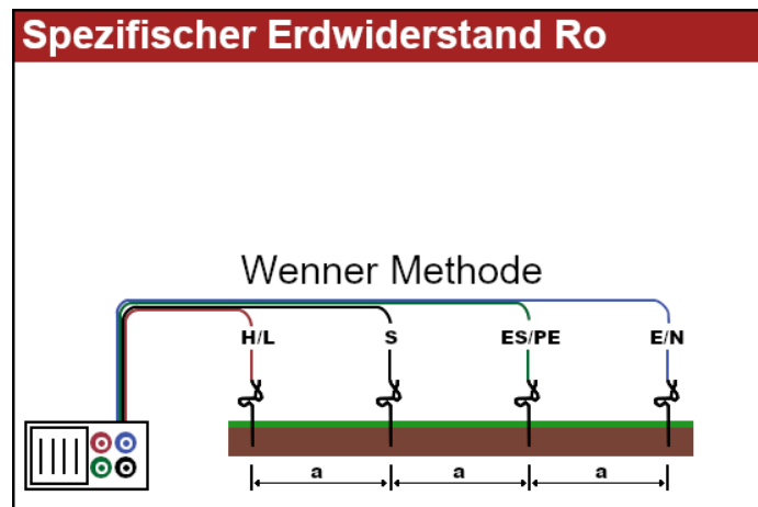
Bild 5.51: Anschlussschema
