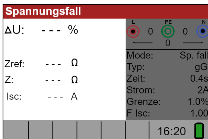
Bild 5.38: Menü Spannungsfallmessung
