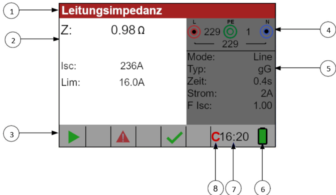
Bild 3.5: Typisches Funktionsdisplay
