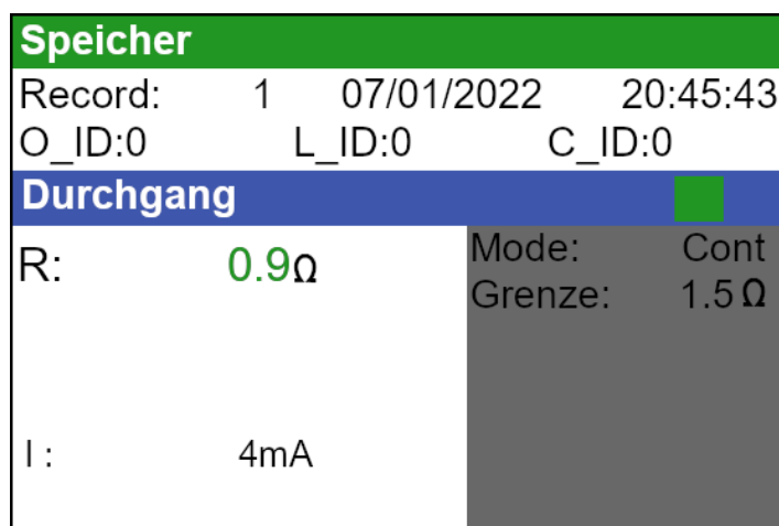
Bild 8.6: Gespeicherte Ergebnisse
