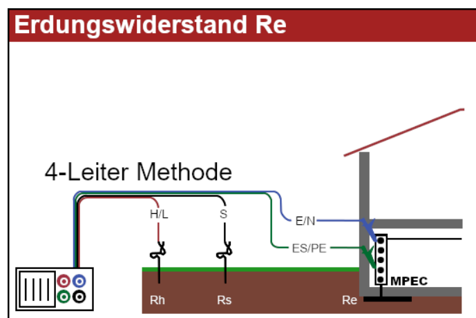
Bild 5.47: 4-Leiter-Anschlussschema
