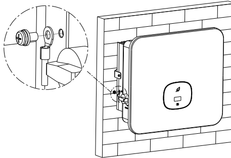
Abb. 6.1 Erdungsschema
