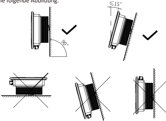
Abb. 5.1 Installationschema
