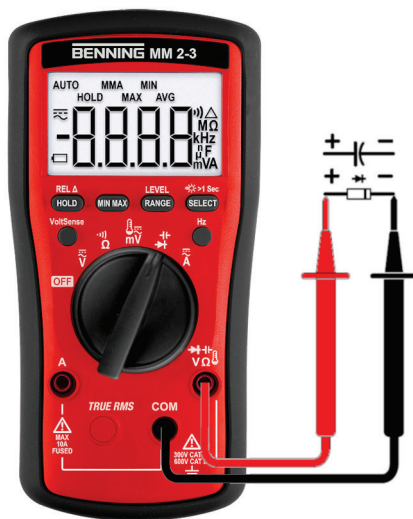
Abb. 12: Kapazitätsmessung oder Diodenprüfung
