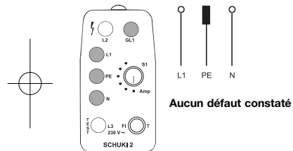
Figure 2 : toutes les lampes de la zone jaune s'allument. En touchant l'électrode, la lampe GL1 doit s'allumer.
