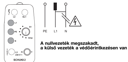
9. ábra: Az L1 , PE és N lámpa világít. Az elektróda érintése nem vált ki hatást.
