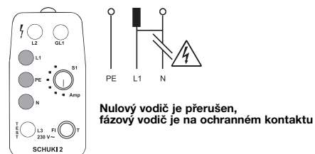
Obrázek 9: Svítí signálky L1 , PE a N . Žádná reakce při dotyku elektrody.
