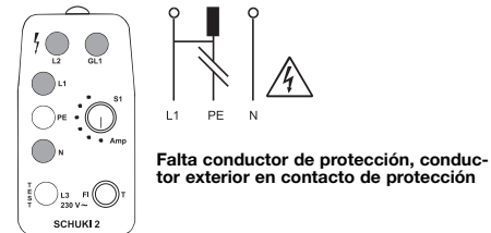
Figura 8: Se iluminan las lámparas N, L1 y L2. GL1 se ilumina al tocar el electrodo.
