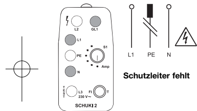
Bild 6: Die Lampen L1 und N leuchten. GL1 leuchtet beim Berühren der Elektrode.
