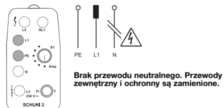
Ilustr. 5: Lampki L1 i PE świecą się. Brak reakcji przy dotknięciu elektrody.
