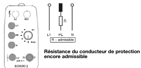
Figure 11 : toutes les lampes de la zone jaune sont allumées. L3 s'allume en plus à l'appui sur la touche T , PE s'éteint simultanément. Après le déclenchement du circuit de protection différentielle, toutes les lampes s'éteignent. Le conducteur de protection possède une résistance plus élevée mais encore admissible.
