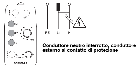
Figura 9: Le spie L1, PE e N si accendono. Nessun effetto a contatto dell'elettrodo.
