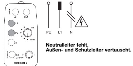
Bild 5: Die Lampen L1 und PE leuchten. Keine Wirkung beim Berührung der Elektrode.
