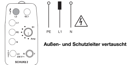
Bild 7: Nur die Lampe L2 leuchtet. Das Berühren der Elektrode hat keine Wirkung.
