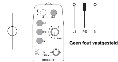
Afbeelding 2: Alle lampjes in het gele gebied branden. Bij aanraking van de electrode moet lampje GL1 gaan branden.
