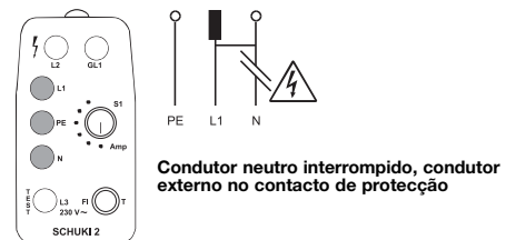
Fig 9: As lâmpadas L1, PE e N acendem. Não há qualquer efeito ao tocar no eléctrodo.
