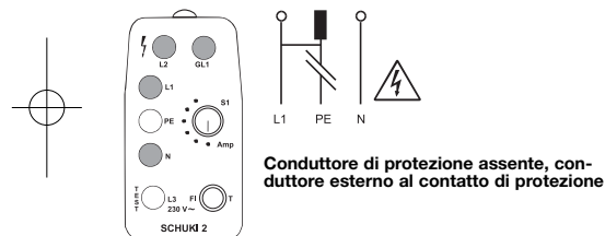
Figura 8: Le spie N, L1 e L2 si accendono. La spia GL1 si accende al contatto dell'elettrodo.
