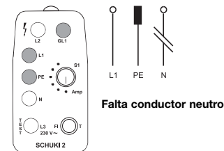
Figura 4: Se iluminan las lámparas L1 y PE . GL1 se ilumina al tocar el electrodo.
