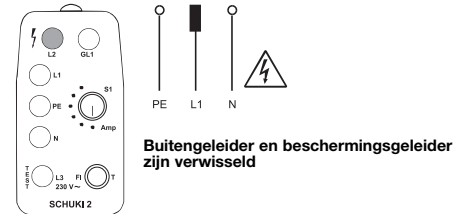
Afbeelding 7: Alleen lampje L2 brandt. Geen effect bij aanraking van de electrode.
