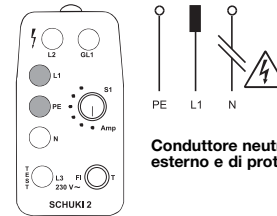
Figura 5: Le spie L1 e PE si accendono. Nessun effetto a contatto dell'elettrodo.
