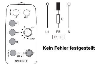
Bild 10: Alle Lampen im gelben Bereich leuchten. Die Lampe L3 leuchtet zusätzlich beim Drücken der Taste T auf. Nach dem Auslösen der FI-Schutzschaltung erlöschen alle Lampen.
