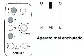
Figura 3: Se iluminan las lámparas N , L1 y L2 . Al tocar el electrodo no se ilumina GL1 .
