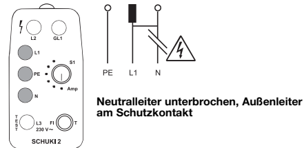
Bild 9: Die Lampen L1 , PE und N leuchten. Keine Wirkung beim Berühren der Elektrode.
