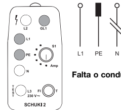
Fig 4: As lâmpadas L1 e PE acendem. A GL1 acende ao tocar no eléctrodo.
