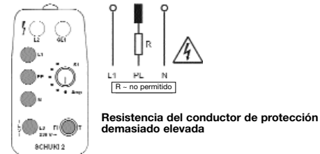
Figura 12: Se iluminan todas las lámparas en la sección amarilla. L3 se ilumina adicionalmente al pulsar la tecla T . Al mismo tiempo se apaga PE y L2 se ilumina brevemente.
