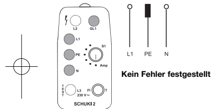
Bild 2: Es leuchten alle Lampen im gelben Bereich. Beim Berühren der Elektrode muss die Lampe GL1 leuchten.
