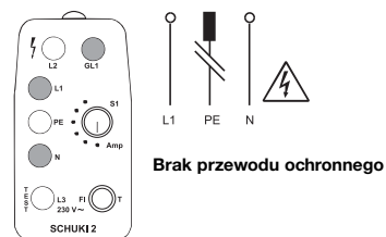
Ilustr. 6: Lampki L1 i N świecą się. GL1 świeci się przy dotknięciu elektrody.
