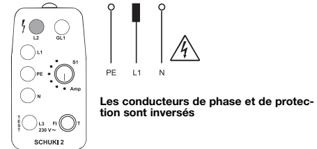
Figure 7 : Seule la lampe L2 s'allume. Toucher l'électrode ne produit aucun effet.
