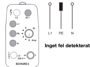
Bild 2: Alla lampor i det gula området lyser. Vid beröring av elektroden måste GL1 lampen lysa.
