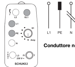
Figura 4: Le spie L1 e PE si accendono. La spia GL1 si accende al contatto dell'elettrodo.
