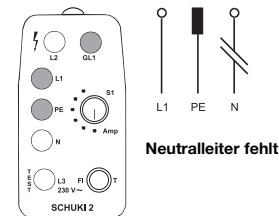
Bild 4: Die Lampen L1 und PE leuchten. GL1 leuchtet beim Berühren der Elektrode.
