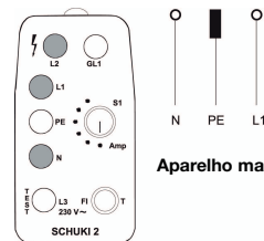
Fig 3: As lâmpadas N , L1 e L2 acendem. Ao tocar no eléctrodo, a GL1 não acende.
