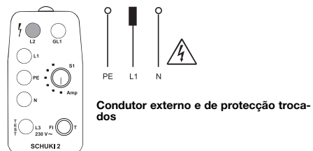
Fig 7: Só acende a lâmpada L2 . Não há qualquer efeito ao tocar no eléctrodo. Esta figura de erro também surge quando o aparelho de teste está mal ligado.
