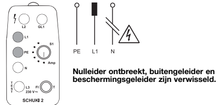
Afbeelding 5: De lampjes L1 en PE branden. Geen effect bij aanraking van de electrode.
