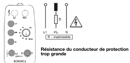
Figure 12 : toutes les lampes de la zone jaune sont allumées. L3 s'allume en plus en appuyant sur la touche T . Simultanément, PE s'éteint et L2 clignote un bref instant. Au bout de 200 ms L3 s'éteint, les lampes en zone jaune restent allumées. La protection différentielle ne déclenche pas. Le conducteur de protection a une résistance élevée inadmissible. Des tensions élevées mortelles peuvent s'établir sur le contact de protection !
