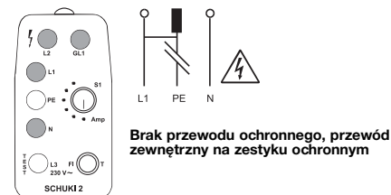
Ilustr. 8: Lampki N, L1 oraz L2 świecą się. GL1 świeci się przy dotknięciu elektrody.
