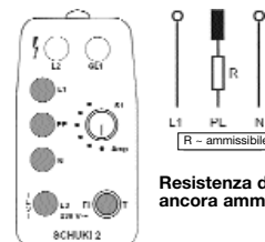
Figura 11: Tutte le spie della zona gialla si accendono.
