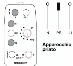
Figura 3: Le spie N , L1 e L2 si accendono. Al contatto dell'elettrodo, la spia GL1 non si accende.
