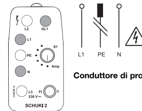
Figura 6: Le spie L1 e N si accendono. La spia GL1 si accende al contatto dell'elettrodo.
