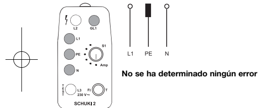
Figura 2: Se iluminan las lámparas en la sección amarilla. Al tocar el electrodo tiene que iluminarse la lámpara GL1 .
