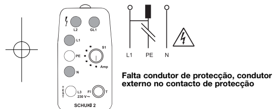
Fig 8: As lâmpadas N, L1 e L2 acendem. GL1 acendem ao tocar no eléctrodo.
