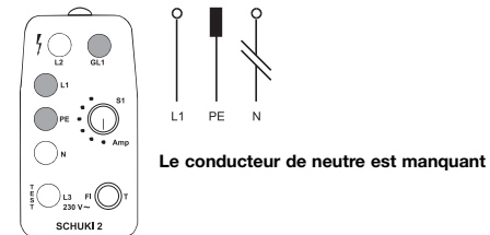
Figure 4 : Les lampes L1 et PE s'allument. GL1 s'allume quand on touche l'électrode.
