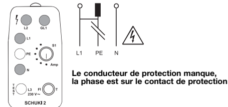
Figure 8 : Les lampes N, L1 et L2 s'allument. GL1 s'allume quand on touche l'électrode.
