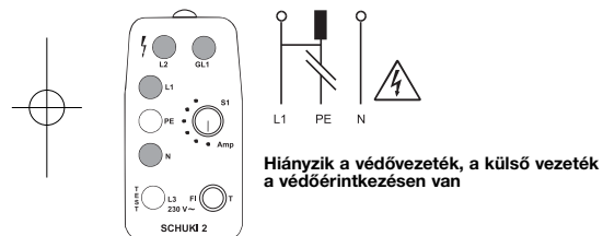
8. ábra: Az N , L1 és L2 lámpák világítanak. Az elektróda megérintésekor GL1 világít.
