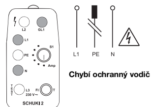
Obrázek 6: Svítí signálky L1 a N . Při dotyku elektrody GL1 svítí. Fázový a ochranný vodič jsou zaměněny.
