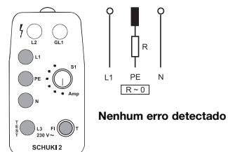
Fig 10: Acendem todas as lâmpadas na zona amarela. A lâmpada L3 acende ainda ao premir a tecla T . Depois de disparar o circuito protector FI, todas as lâmpadas se apagam.
