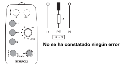
Figura 10: Se iluminan todas las lámparas en la sección amarilla. La lámpara L3 se ilumina adicionalmente al pulsar la tecla T . Después de que haya disparado el interruptor diferencial se apagan todas las lámparas.
