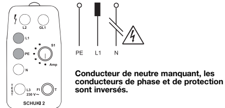
Figure 5 : Les lampes L1 et PE s'allument. Aucun effet quand on touche l'électrode.
