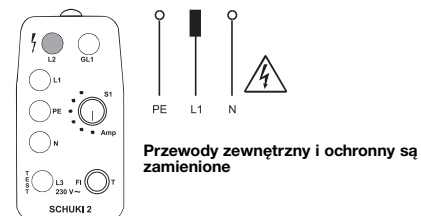
Ilustr. 7: Świeci się tylko lampka L2. Dotknięcie elektrody jest bez skutku.
