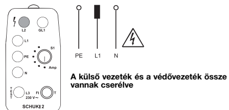
7. ábra: Csak az L2 lámpa világít. Az elektróda érintése nem vált ki hatást.
