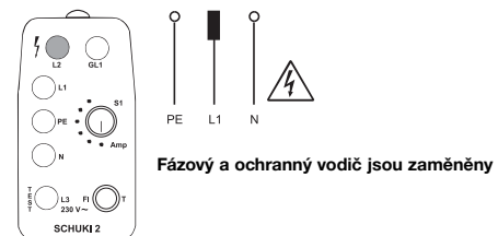
Obrázek 7: Svítí pouze signálka L2 . Žádná reakce při dotyku elektrody.
