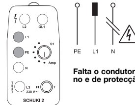
Fig 5: As lâmpadas L1 e PE acendem. Não há qualquer efeito ao tocar no eléctrodo.
