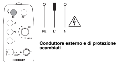
Figura 7: Si accende solo la spia L2. Il contatto dell'elettrodo non sortisce alcun effetto.
