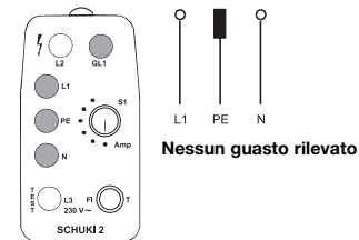
Figura 2: Tutte le spie della zona gialla si accendono. Al contatto dell'elettrodo, la spia GL1 deve accendersi.
