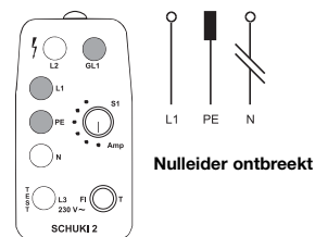
Afbeelding 4: De lampjes L1 en PE branden. GL1 gaat branden bij aanraking van de electrode.
