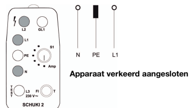
Afbeelding 3: De lampjes N , L1 en L2 branden. Bij aanraken van de electrode gaat GL1 niet branden.
