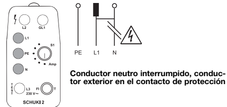
Figura 9: Se iluminan las lámparas L1 , PE y N . No hay efecto alguno al tocar el electrodo.
