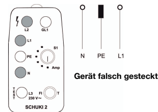
Bild 3: Die Lampen N , L1 und L2 leuchten. Beim Berühren der Elektrode leuchtet GL1 nicht auf.
