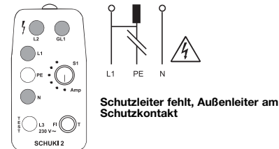
Bild 8: Die Lampen N , L1 und L2 leuchten. GL1 leuchtet beim Berühren der Elektrode.
