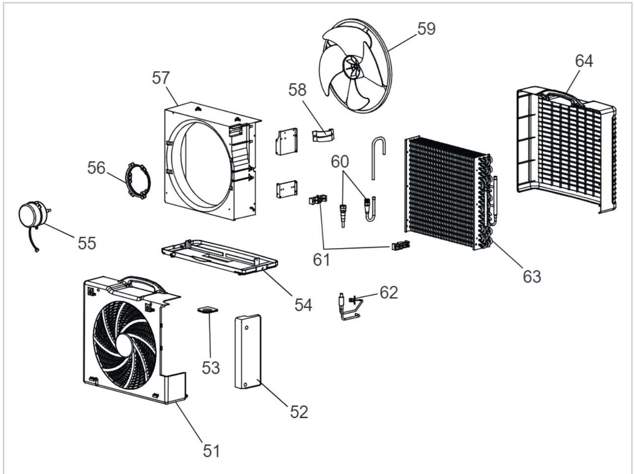
Abb. 19: Explosionszeichnung Außenteil
