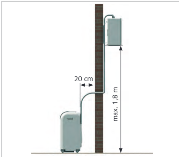
Abb. 10: Maximale Montagehöhe
