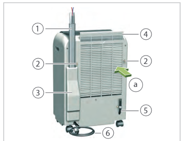
Abb. 2: Rückansicht (Innengerät)
