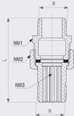
Verschraubung - Rotguss oder Siliziumbronze Modell 3334
