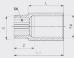
Verlängerung - Rotguss oder Siliziumbronze Modell 3525
