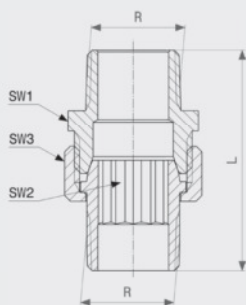
Verschraubung - Rotguss oder Siliziumbronze Modell 3344
