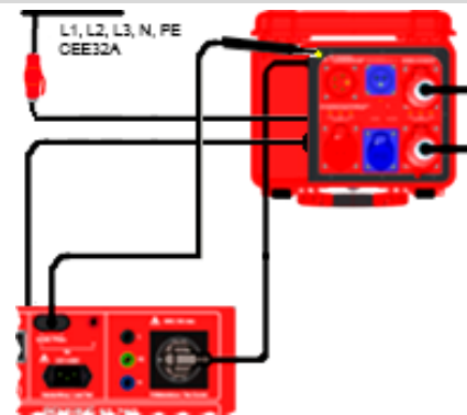
Anschlussschema
