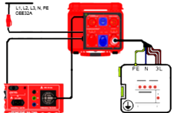
Anschlusschema
