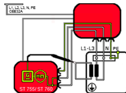
Stromlaufplan
