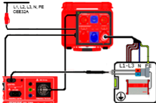
Anschlusschema
